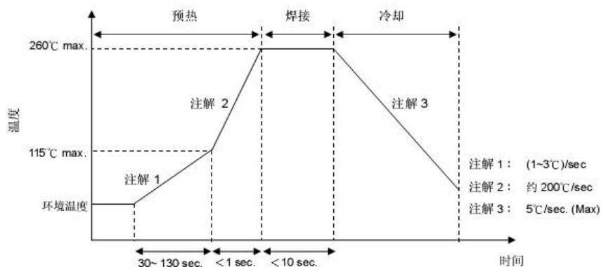
波峰焊曲线
